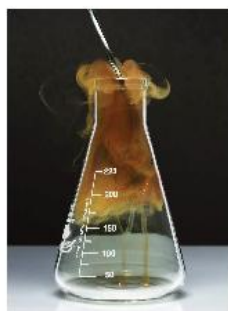
Cl_2 phản ứng với Fe
