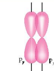
▲ Xen phủ bên pp
