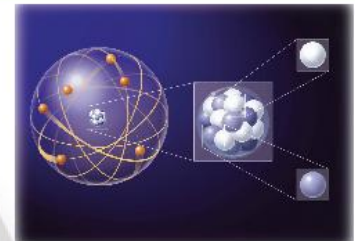
▲ Mô phỏng mô hình nguyên tử
