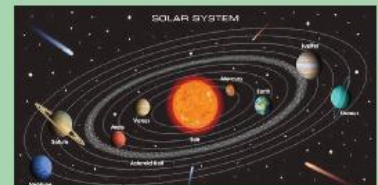
▲ Hệ Mặt Trời
