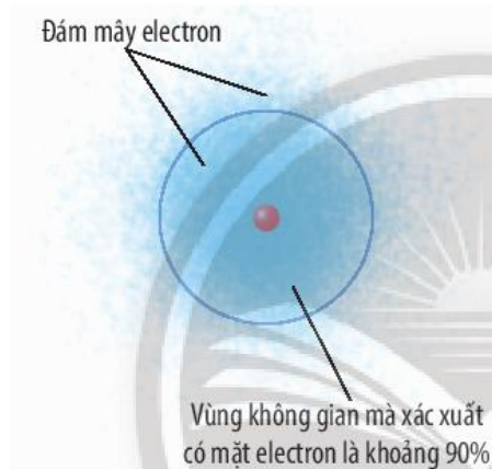
▲ Hình 4.3. Đám mây electron của nguyên tử hydrogen
