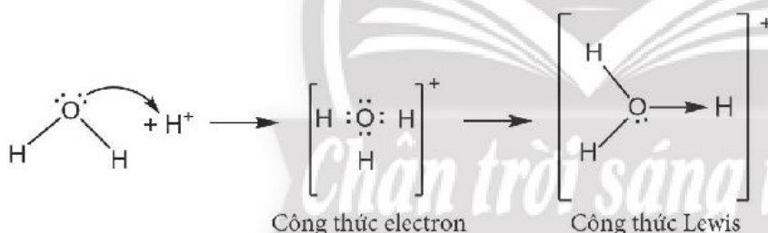
▲ Hình 10.4. Sơ đồ tạo liên kết cho nhận trong ion hydronium \text{H}_3\text{O}^+
