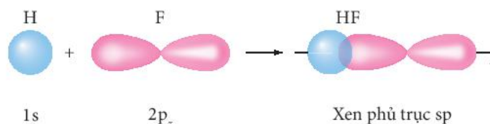
▲ Hình 10.6. Sự xen phủ giữa orbital 1s của nguyên tử hydrogen và orbital 2p của nguyên tử fluorine hình thành liên kết \sigma trong phân tử hydrogen fluoride
