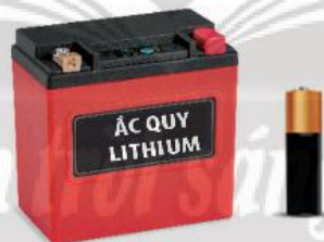
Hình 12.9. Ắc quy và pin
