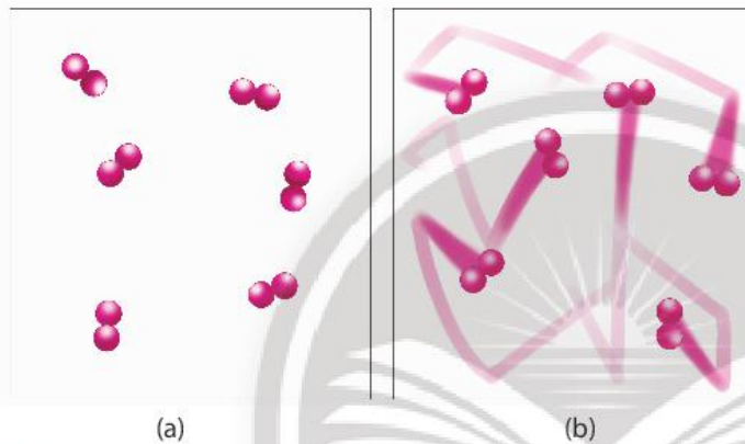
▲ Hình 16.4. Hình minh họa chuyển động của chất phản ứng khi chưa đun nóng (a) và được đun nóng (b)
