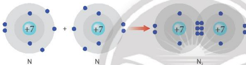
▲ Hình 8.2. Sự hình thành liên kết trong phân tử nitrogen
