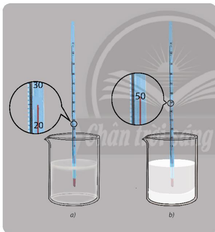
▲ Hình 13.2. Minh hoạ vôi sống phản ứng với nước
