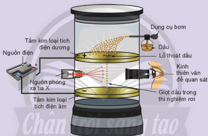
▲ Thí nghiệm giọt dầu của Millikan
