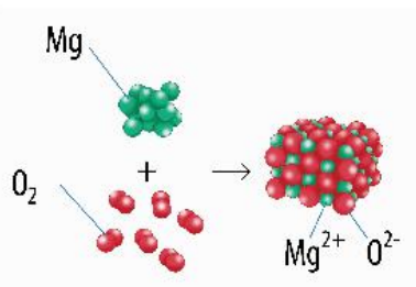
▲ Hình 12.1. Magnesium phản ứng với oxygen
