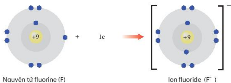
▲ Hình 8.4. Sự hình thành ion F -
