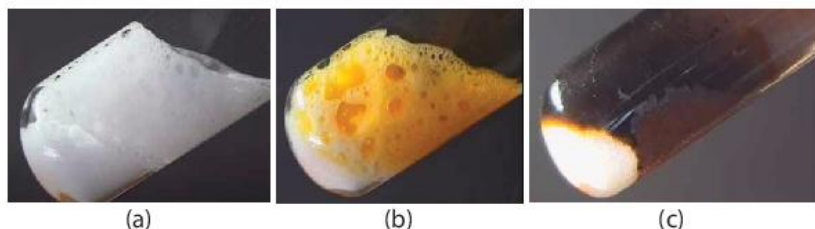
▲ Hình 18.3. Các muối KCl (a), KBr (b), KI (c) phản ứng với dung dịch H_2SO_4 đặc
