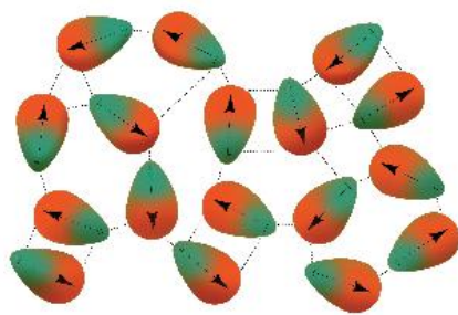
▲ Hình 18.1. Tương tác van der Waals giữa các phân tử HX
