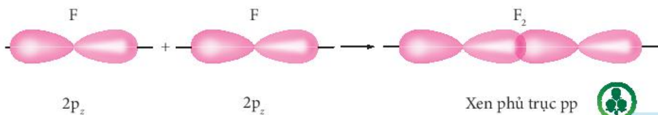
▲ Hình 10.7. Sự xen phủ giữa hai orbital 2p của hai nguyên tử fluorine hình thành liên kết \sigma trong phân tử fluorine
