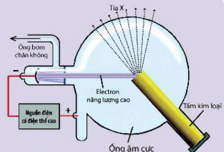
▲ Mô hình thí nghiệm khảo sát bản chất tự nhiên của tia X của Henry Moseley
